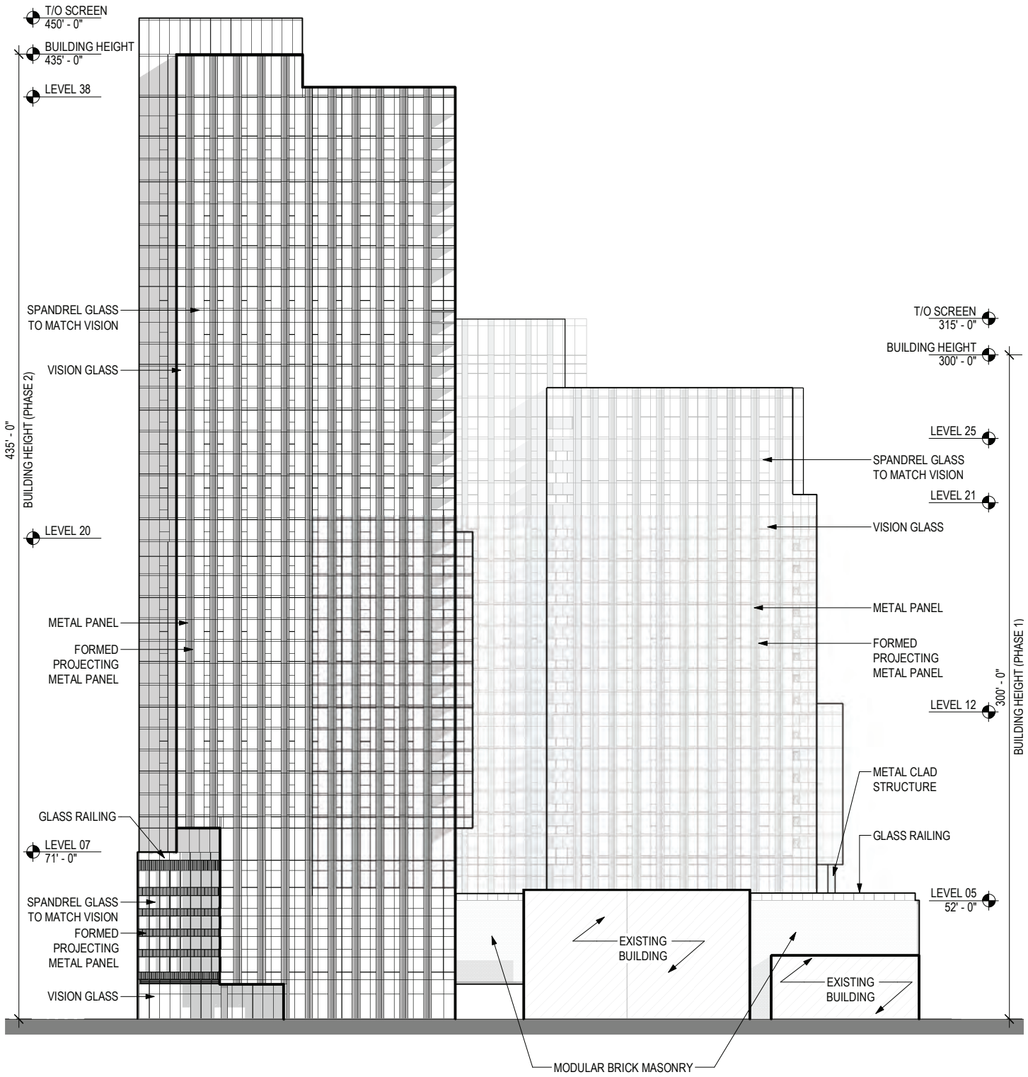
WEST BUILDING ELEVATION Scale: N.T.S.
