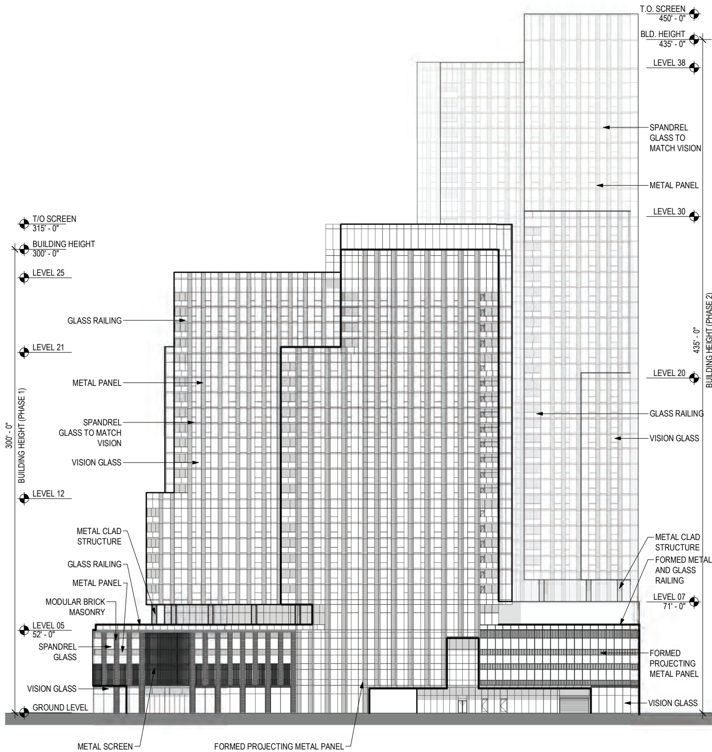
EAST BUILDING ELEVATION Scale: N.T.S.
