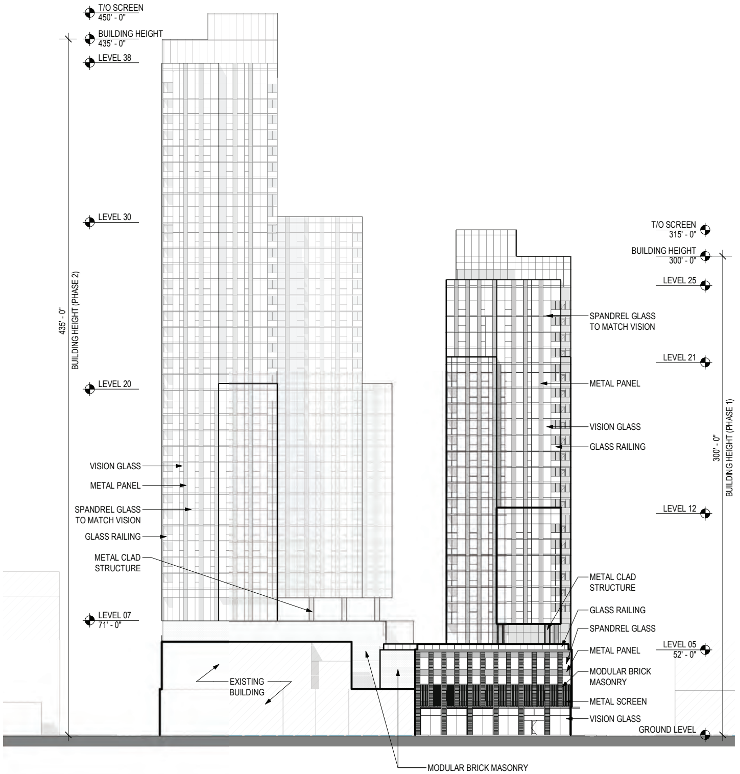
SOUTH BUILDING ELEVATION Scale: N.T.S.
